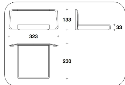
PST (KUSA) KING USA : LETTO PER MATERASSO / BED FOR MATTRESS 195x205 - 323x230x133H. - H.B.33cm 76 2/3x80 2/3 - 127x90 2/3x52 1/3H. - H.B.13"
