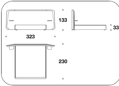
PST (KUSA) KING USA : LETTO PER MATERASSO / BED FOR MATTRESS 195x205 - 323x230x133H. - H.B.33cm 76 2/3x80 2/3 - 127x90 2/3x52 1/3H. - H.B.13"
