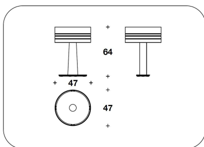
LMB (23) LAMPADA DA TAVOLO / TABLE LAMP Ø 47x64H.cm Ø 18 2/4x25 1/3H."
